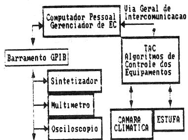
Figura 1: Hardware envolvido na ATE.
